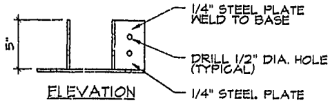
ELEVATION
