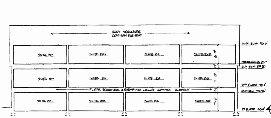
1 THRU SECTION SCALE: 1/8" = 1'-0"
