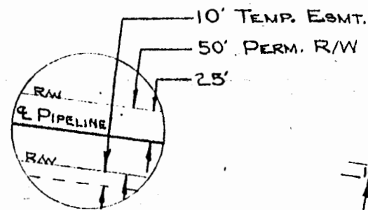
DETAIL "A" SCALE: 1"=100'
