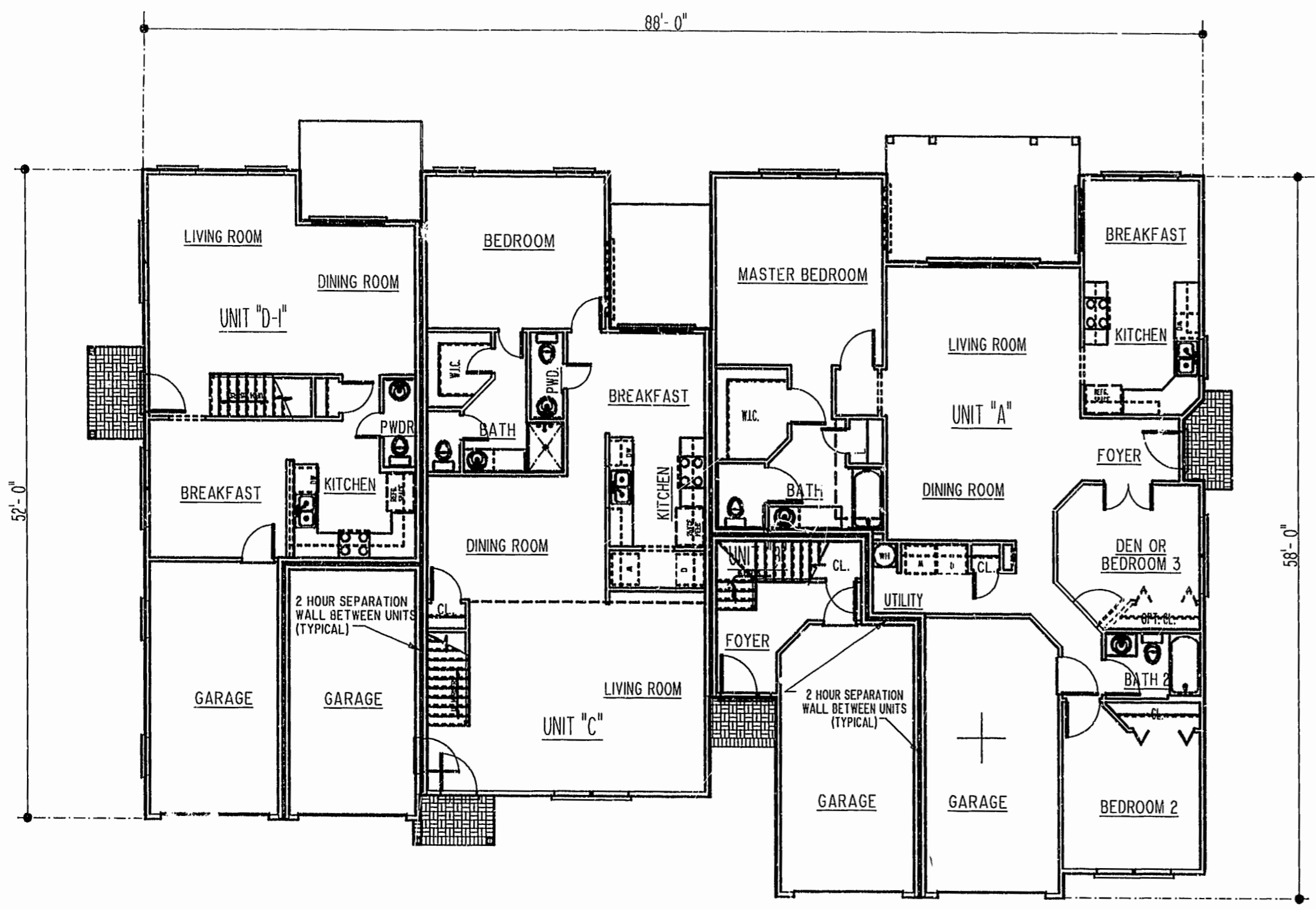
MODEL 400 SCALE: 1/8" = 1'-0"
