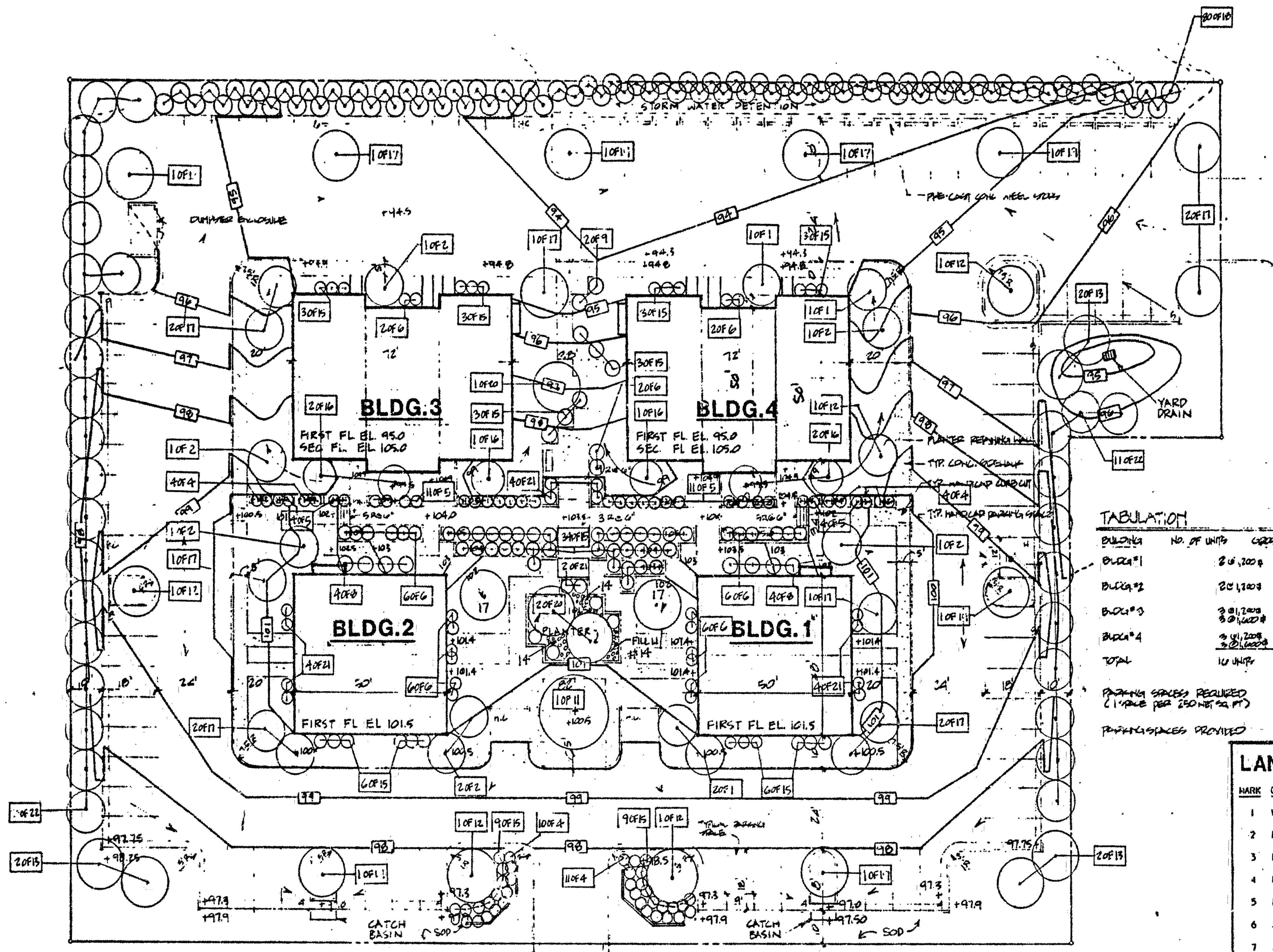
SITE PLAN 1:20
