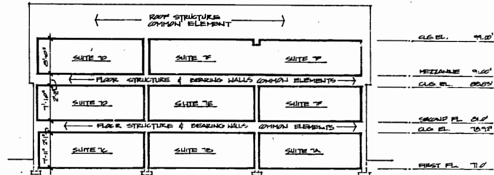
3 THRU SECTION SCALE: 1/8" = 1'-0"
