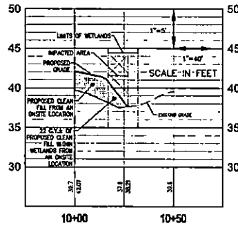
WETLAND IMPACT #1 A-A
