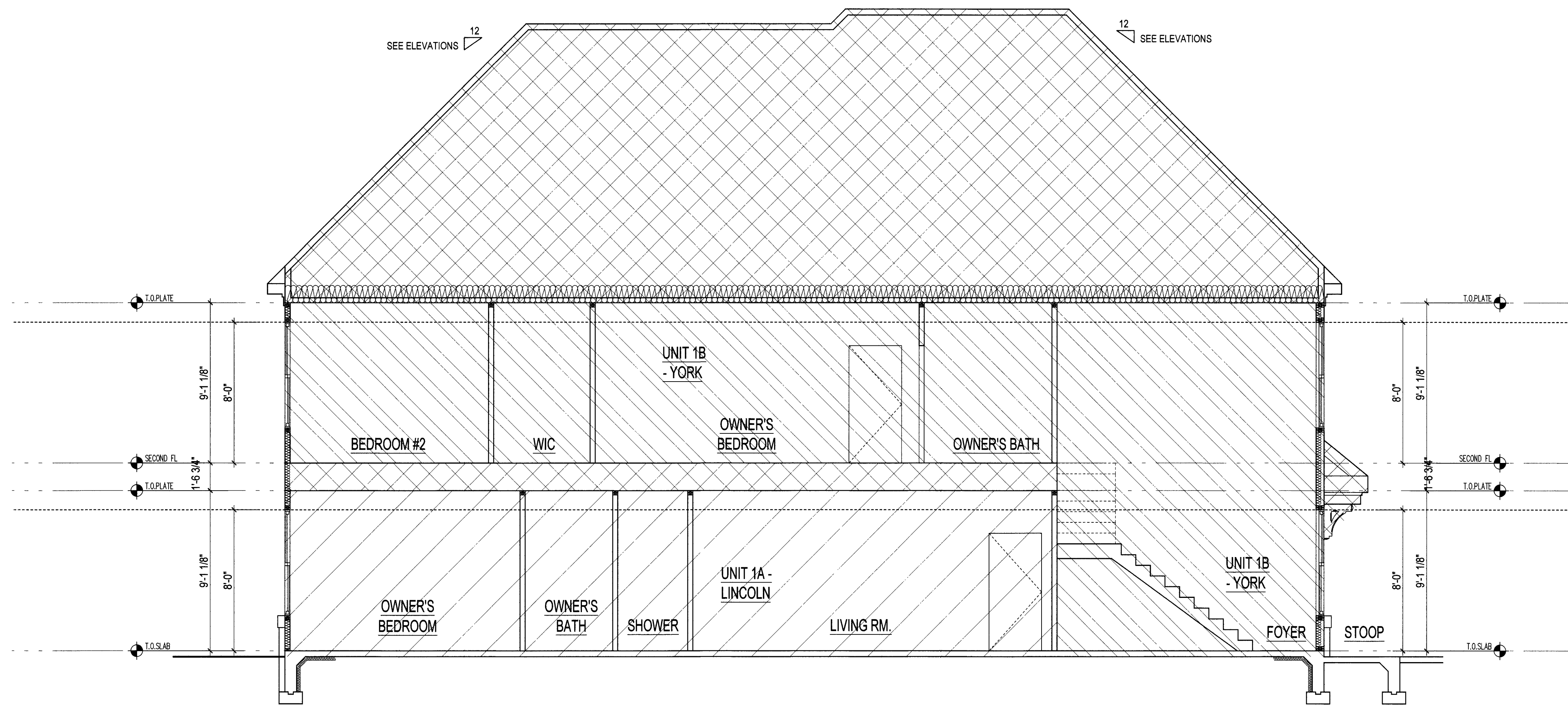
SECTION 1 SCALE: 1/4" = 1'-0" HUN.003A_A4
